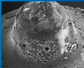
Schmutzablagerung auf einer vergrößerten Einspritzdüse eines Dieselmotors.
